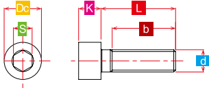
CAP BOLT M6 P=1.0 L 10 mm - 45 mm
